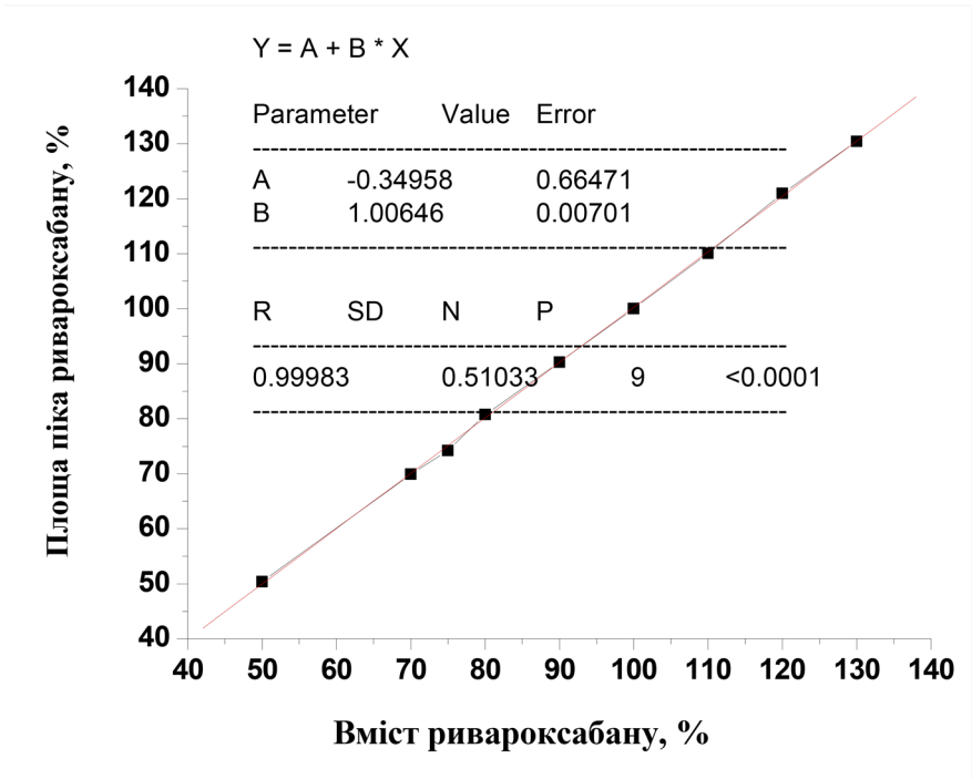
Рис. 3. Лінійна залежність площі піка від концентрації в нормалізованих координатах для визначення ривароксабану
