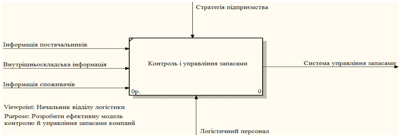
Рис. 35. Контекстна діаграма
