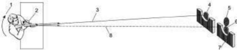
Іл. 21.3. Уточнення наведення гвинтівки по горизонталі під час стрільби сидячи за столом: 1 — напрямок повороту корпусу стрільця; 2 — вісь обертання корпусу стрільця; 3 — лінія прицілювання до уточнення наведення гвинтівки; 4 — точка наведення гвинтівки до уточнення наведення; 5 — «яблучко» мішені — виявилось праворуч; 6 — точка наведення та прицілювання; 7 — розташування прицілу після уточнення наведення гвинтівки; 8 — лінія прицілювання після уточнення наведення гвинтівки
