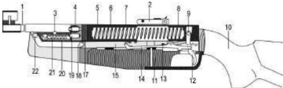
Іл. 20.4. Складові частини і механізми рушниць ДК-38: 1 — ствол; 2 — приціл; 3 — вісь ствола; 4 — прокладка ствола; 5 — коробка ствола; 6 — поршень; 7 — пружина бойова; 8 — колодка механізму спускового; 9 — штифт колодки; 10 — ложа; 11 — гвинт ложі задній; 12 — гачок спусковий; 13 — шептало; 14 — важіль блокування; 15 — важіль зведення; 17 — манжета; 18 — шарнір; 19 — клин; 20 — ригель; 21 — пружина ригеля; 22 — вісь шарніра
