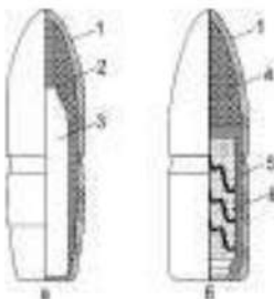
Іл. 22.4. Куля: а — звичайна зі сталевим осердям; б — трасуюча; 1 — оболонка; 2 — свинцева сорочка; 3 — сталеві серцевина; 4 — свинцева серцевина; 5 — стаканчик трасера; 6 — трасуюча суміш
