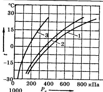
Рис. 32. Графік залежності тиску насичених парів ядучих речовин від температури: 1 — аміак; 2 — хлор; 3 — сірчангий ангідрид
