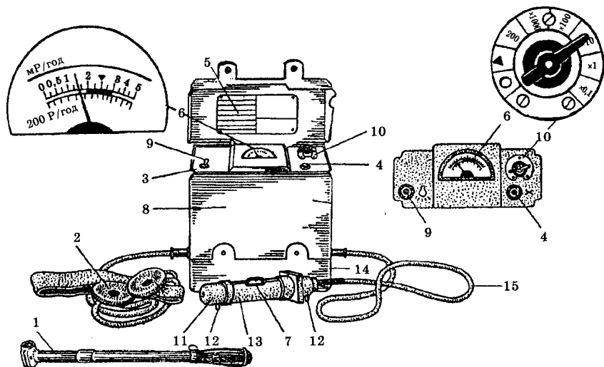
Рис. 11. Прилад ДП-5В:
