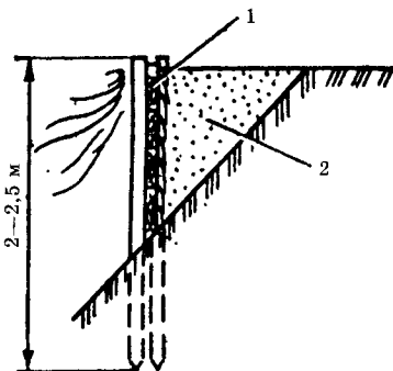
Рис. 2. Дощата стінка:
