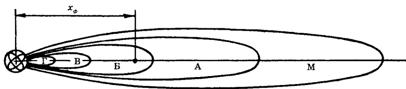
Рис. 27. Визначення дози опромінення при перебуванні на осі хмари радіоактивного забруднення після аварії на АЕС
