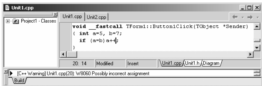
Рис. 14.27. Попередження W8060: замість операції порівняння використано оператор присвоювання
