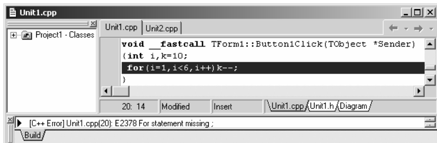
Рис. 14.23. Помилка E2378: розділювач у операторі for – кома замість крапки з комою
