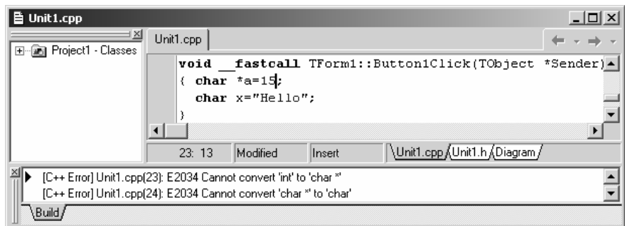
Рис. 14.17. Помилка E2034: суперечка типів
