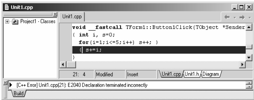
Рис. 14.18. Помилка E2040: фігурна дужка закрита завчасно
