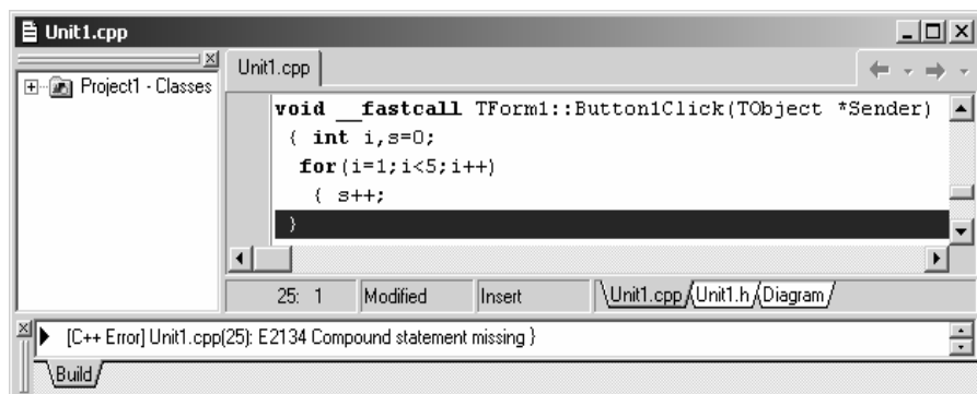
Рис. 14.10. Помилка E2134: пропущено закрити фігурну дужку
