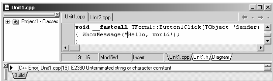
Рис. 14.21. Помилка E2380: пропущено лапки
