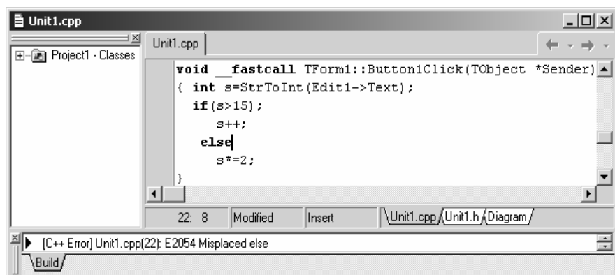
Рис. 14.15. Помилка E2054: неможливо встановити, до якого if належить else , через зайву крапку з комою після умови
