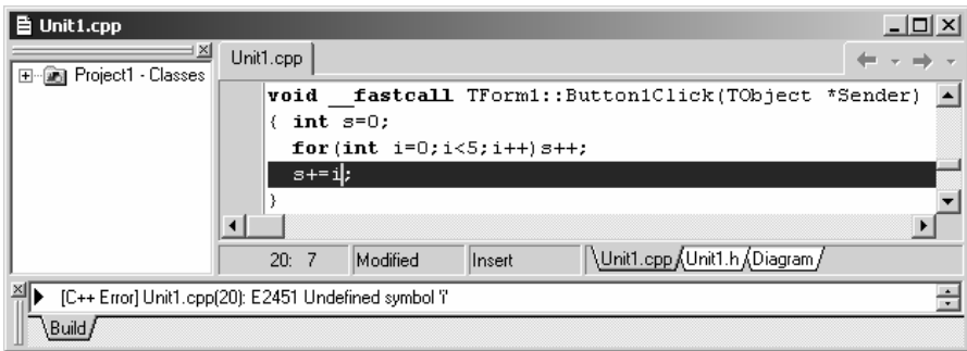
Рис. 14.8. Помилка E2451: змінну i оголошено в іншій області видимості
