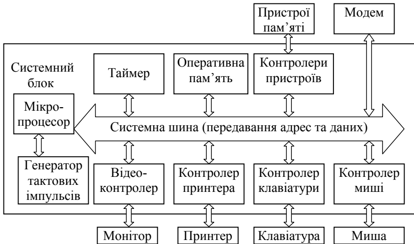
Рис. 1.1. Типова архітектура комп'ютера
