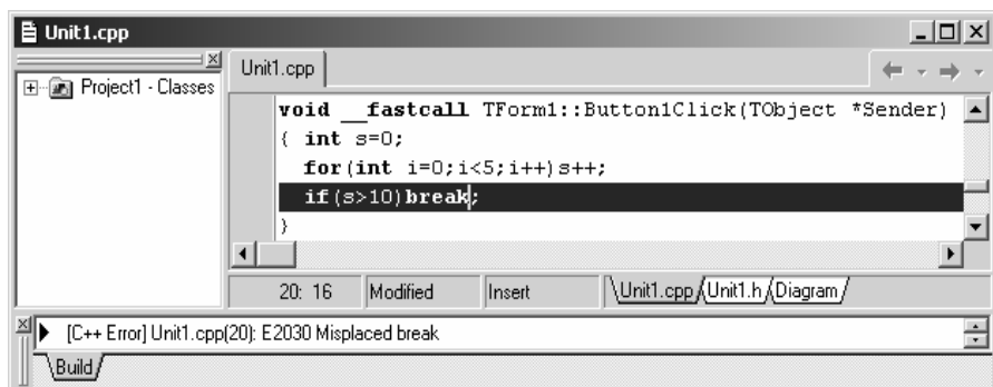
Рис. 14.14. Помилка E2030: пропущено фігурні дужки і вживання break немає сенсу
