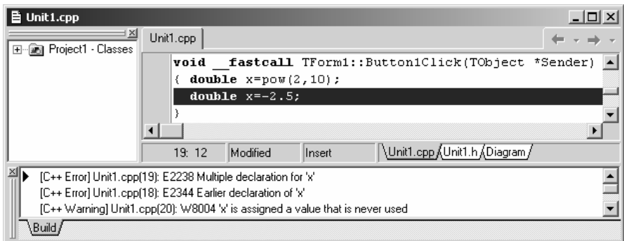
Рис. 14.9. Помилка E2238: змінну x оголошено двічі
