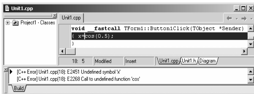
Рис. 14.7. Помилка E2451: не оголошено змінну x
