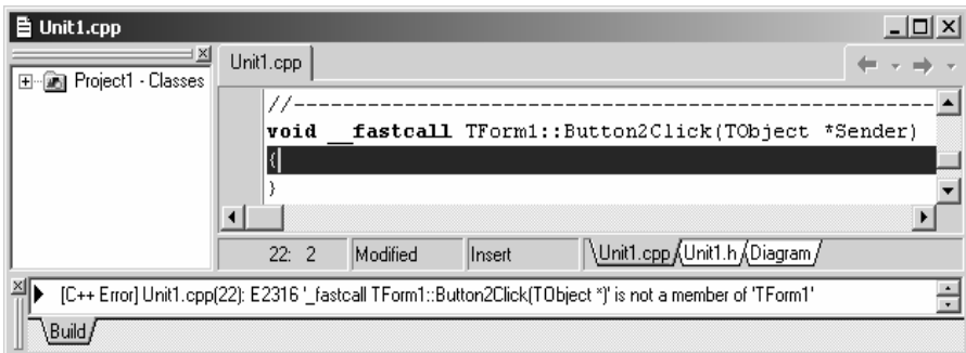
Рис. 14.5. Помилка E2316: заголовок відгуку на подію написано власноруч
