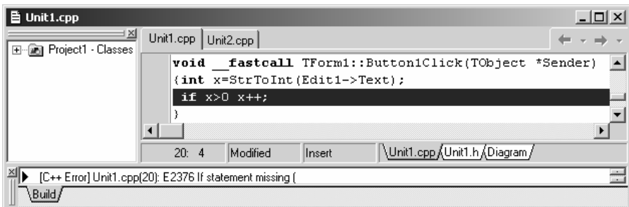
Рис. 14.22. Помилка E2376: пропущено дужки в умові оператора if
