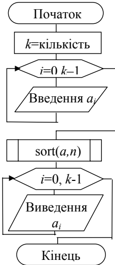
Схема алгоритму до основної програми
