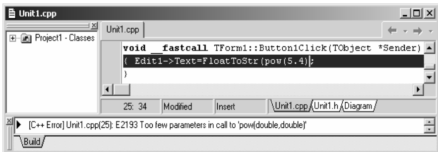
Рис. 14.13. Помилка E2193: виклик функції pow() з одним параметром замість двох
