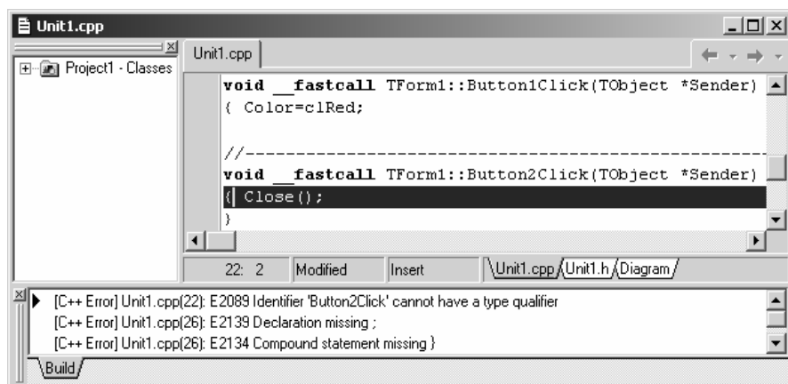
Рис. 14.6. Помилка E2089: пропущено закрити дужку у попередній функції
