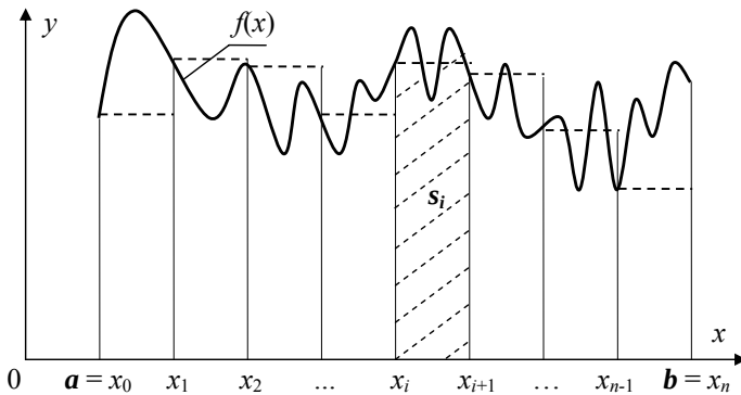
Рис. 4.2. Інтерпретація інтегрування методом прямокутників
