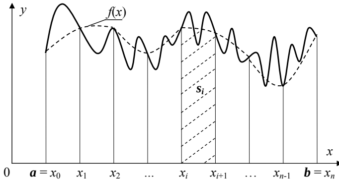
Рис. 4.4. Інтерпретація інтегрування методом Сімпсона
