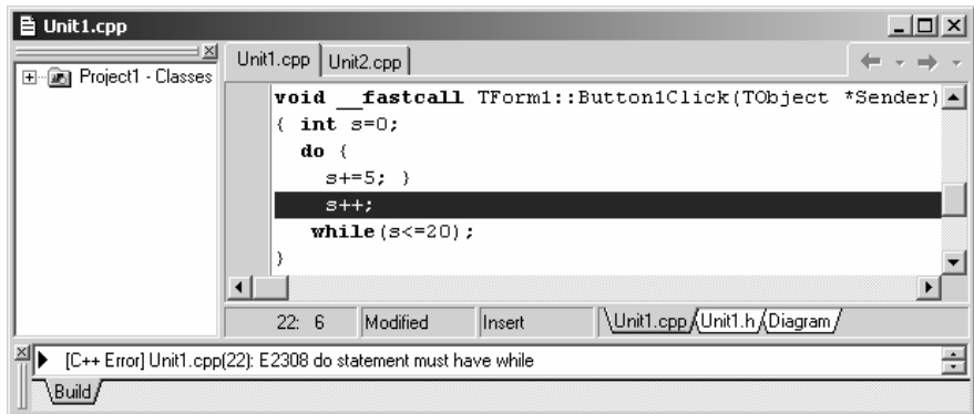
Рис. 14.20. Помилка E2308: завчасно закрито фігурну дужку
