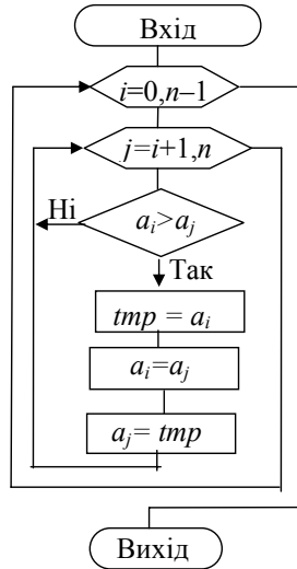
Схема алгоритму функції sort()
