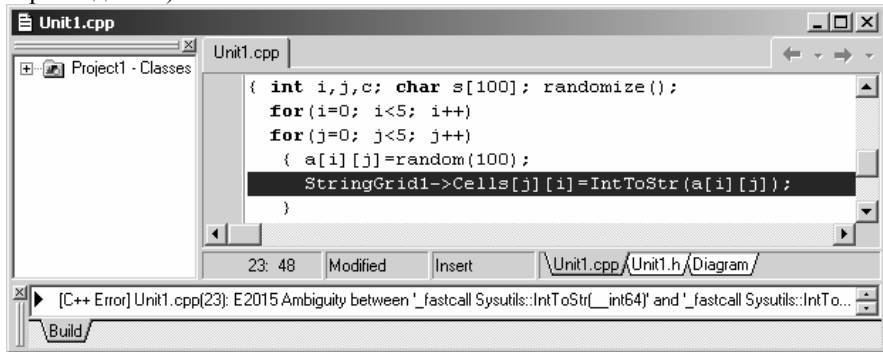
Рис. 14.26. Помилка E2378: фактичний параметр у функції IntToStr() дійсний замість цілого
