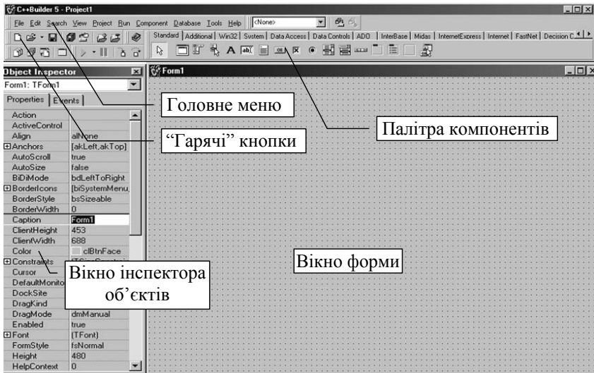
Рис. 2.1. Вигляд головного вікна середовища C++ Builder
