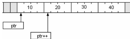
Рис. 6.1. Операція інкремента покажчика
