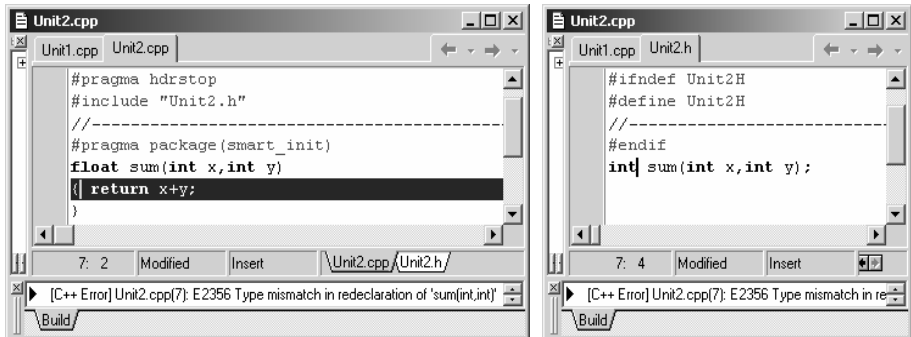
Рис. 14.19. Помилка E2356: типи функції в оголошенні та визначенні не збігаються
