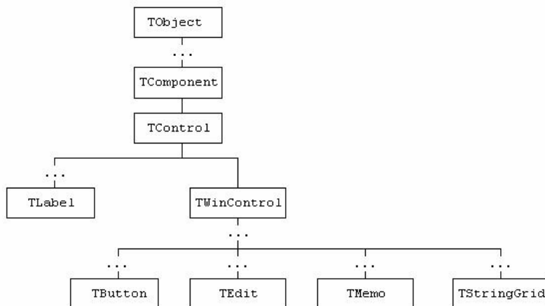
Рис. 13.1. Ієрархія класів бібліотеки VCL
