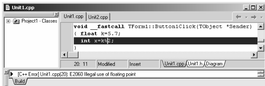
Рис. 14.25. Помилка E2378: операцію обчислення остачі від ділення дійсних чисел не визначено
