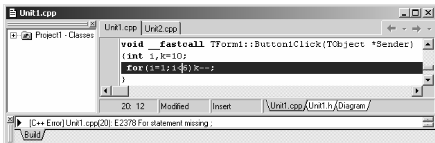
Рис. 14.24. Помилка E2378: друга крапка з комою у for є відсутня
