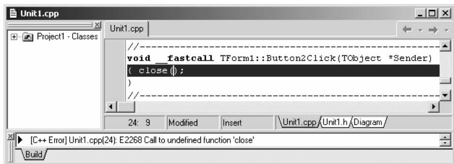
Рис. 14.3. Помилка E2268: ім'я функції написано неправильно
