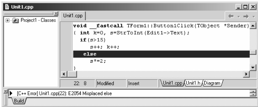
Рис. 14.16. Помилка E2054: неможливо встановити, до якого if належить else, через те, що пропущено фігурні дужки
