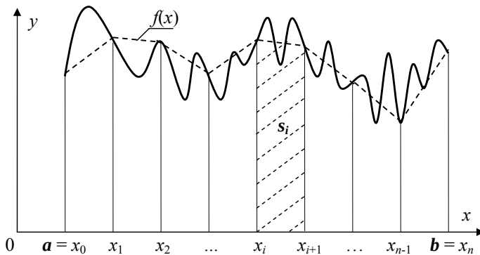
Рис. 4.3. Інтерпретація інтегрування методом трапецій
