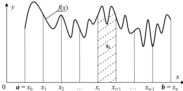
Рис. 4.1. Криволінійні трапеції для інтегрування
