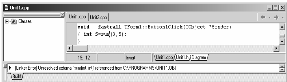
Рис. 14.28. Помилка на етапі компонування: імена функції в оголошенні (у .h файлі) та визначенні (у .cpp файлі) не збігаються
