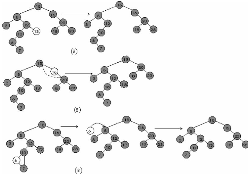
Рис. 12.2. Різні випадки вилучення вузлів дерева:
