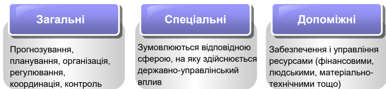
Рис.4.1 Функції управління
